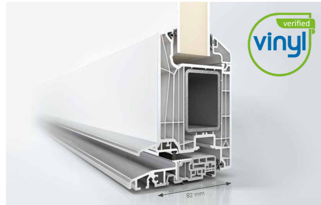
Schüco LivIng Système de porte d'entrée PVC
